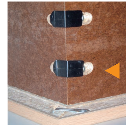
snelle montage van het kozijn door het gebruik van een klips-schroef verbinding
